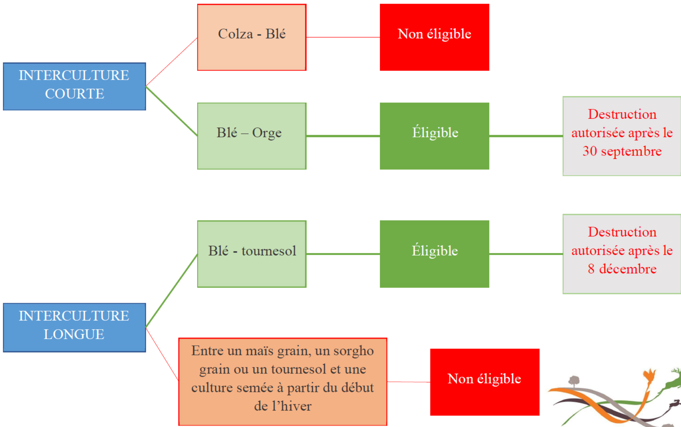
Schéma d'éligibilité à la subvention « Maintien des chaumes » par la Fédération des chasseurs de la Vienne
